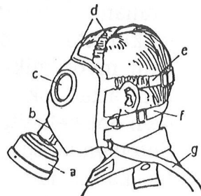
Kaasunaamari. a suodatin, b leuka-kappale, c naamarilasit, d, e ja / kiinnitysnauhasto, g kantohihna.
